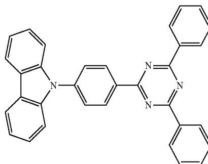
DPEPO
