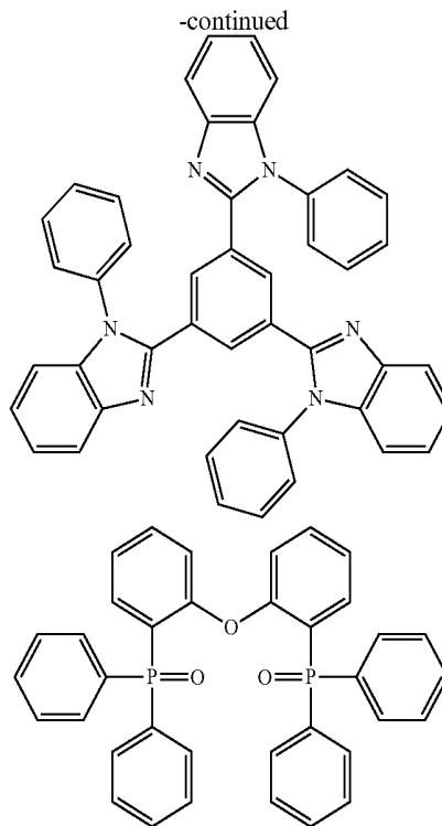
DPEPO
